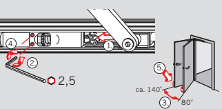
Openhoudpositie instellen
