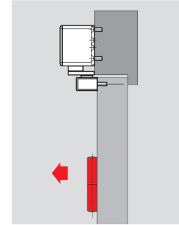
Kozijndorpelmontage scharnierzijde
