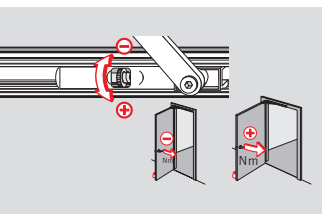
Uittrekkraft instellen
