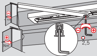
Uittrekkraft instellen
